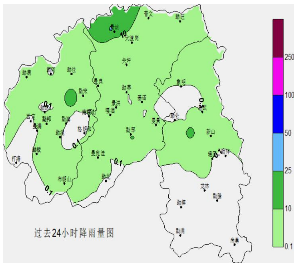
图1 西双版纳州7月26日08时~27日08时降雨量图(单位:毫米)
